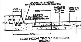
GUARNICION TIPO "L" (BO 15/m) EN SECA
