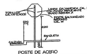
POSTE DE ACERO
